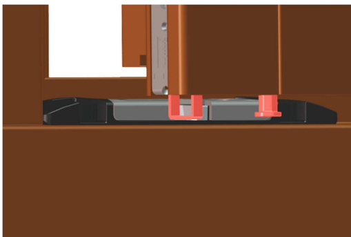
Das Fenster ist offen und die Zusatzverriegelung geöffnet.
