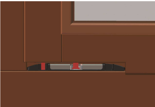
Das Fenster ist geschlossen, jedoch noch nicht durch die Zusatzverriegelung gesichert.
